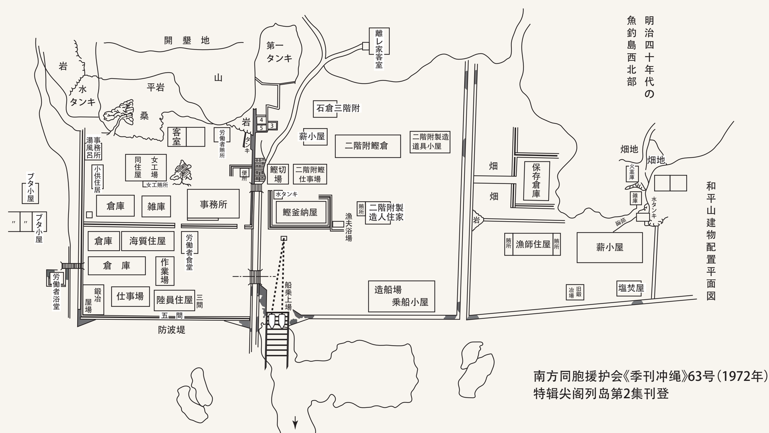
鱼钓岛事业所建筑物布局图（明治40年代，古贺辰四郎制作）
