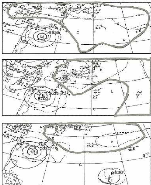
第2図 500hPa実況図(色塗りが太平洋高気圧) 上から台風第5号、9号、13号の接近時(15号は省略)
