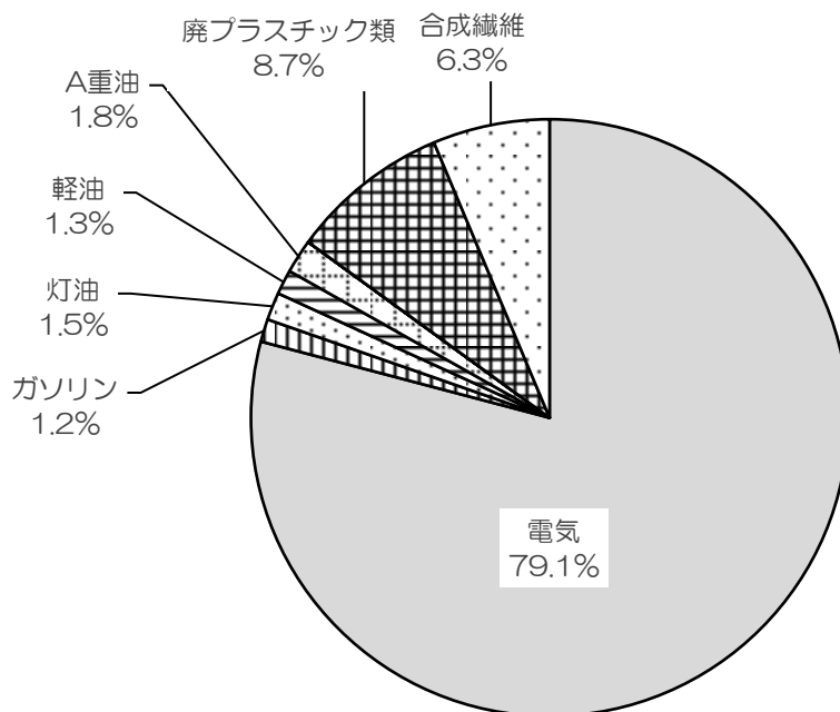
図 3-2 発生源別二酸化炭素排出割合
