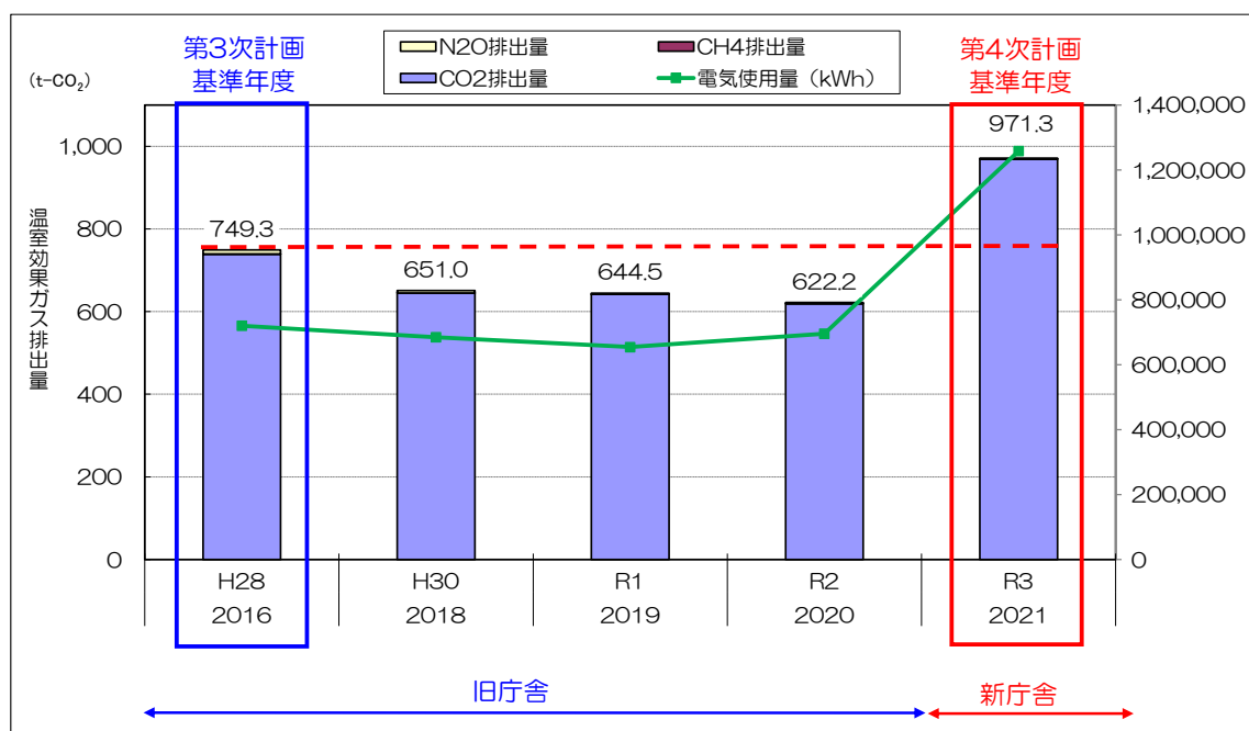
図3-5 本市の温室効果ガス排出量の推移
