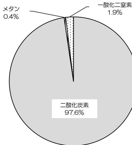
図 3-1 基準年（令和3年度）温室効果ガス排出割合
