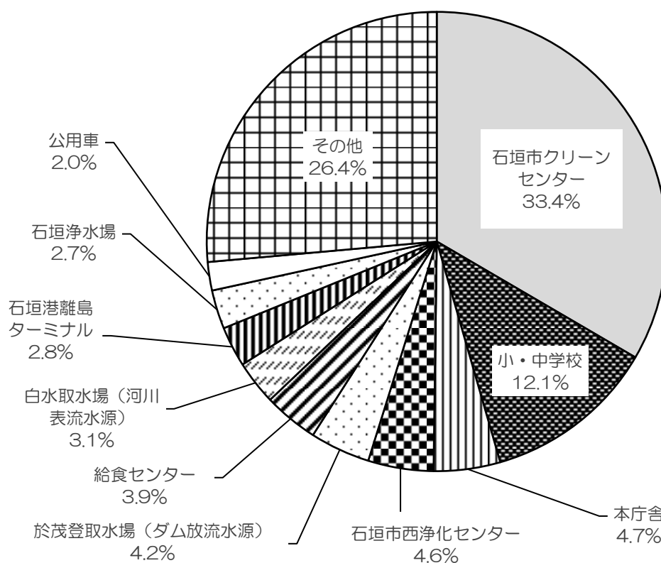
図 3-4 施設別温室効果ガス排出割合
