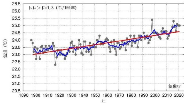
図1-3 石垣島の年平均気温の経年変化
