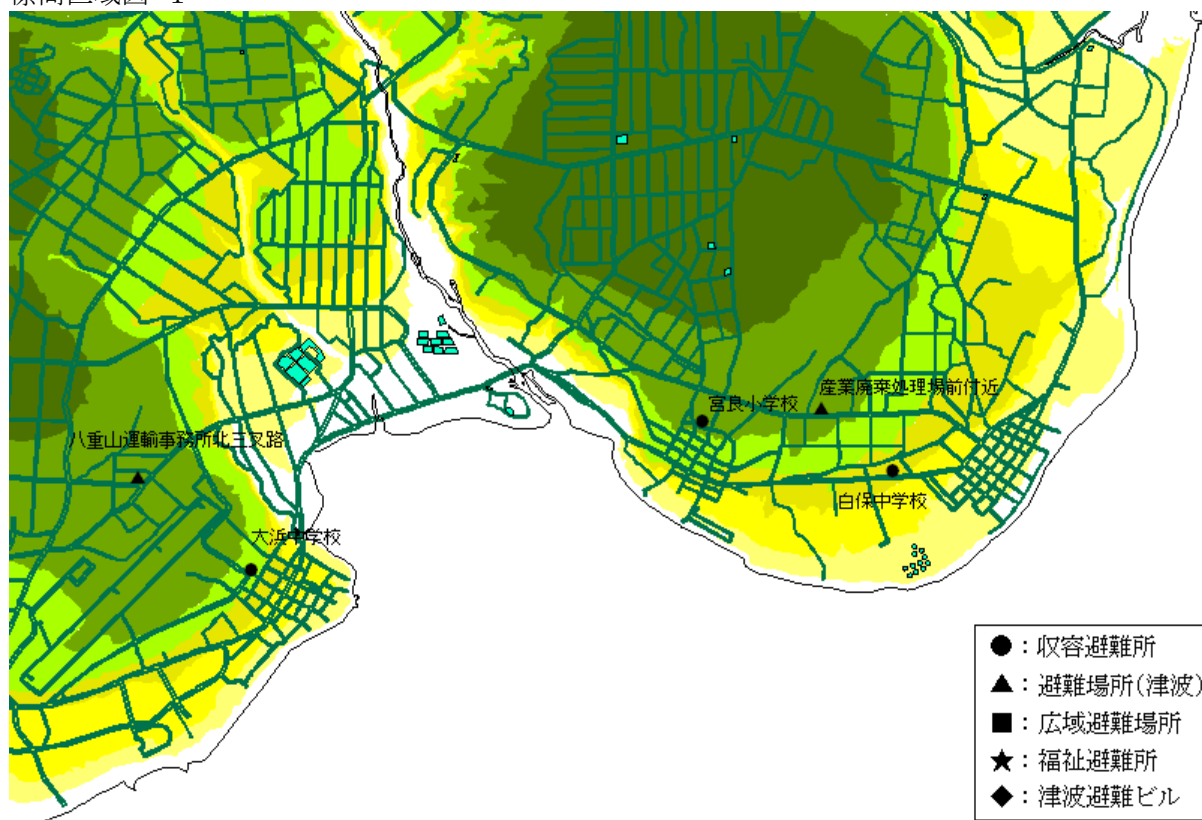
標高区域図 1
