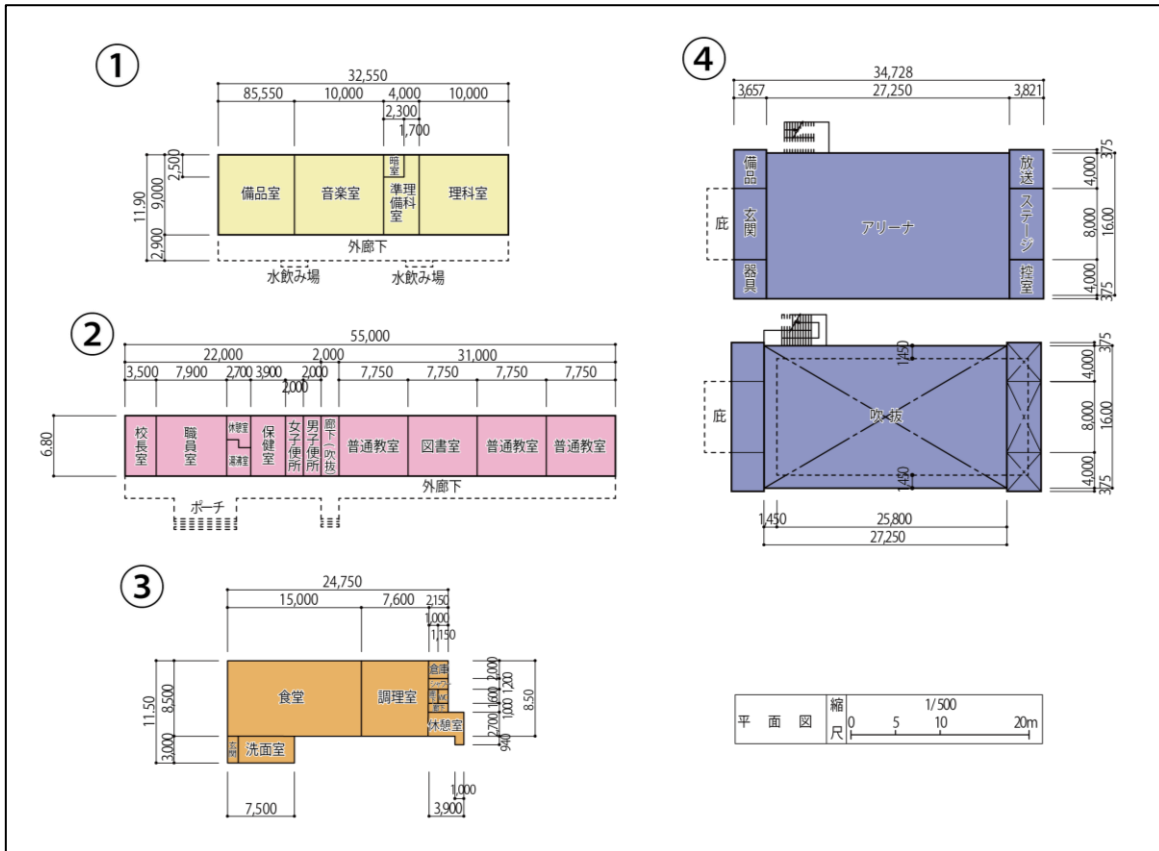
図 28. 施設の平面図
