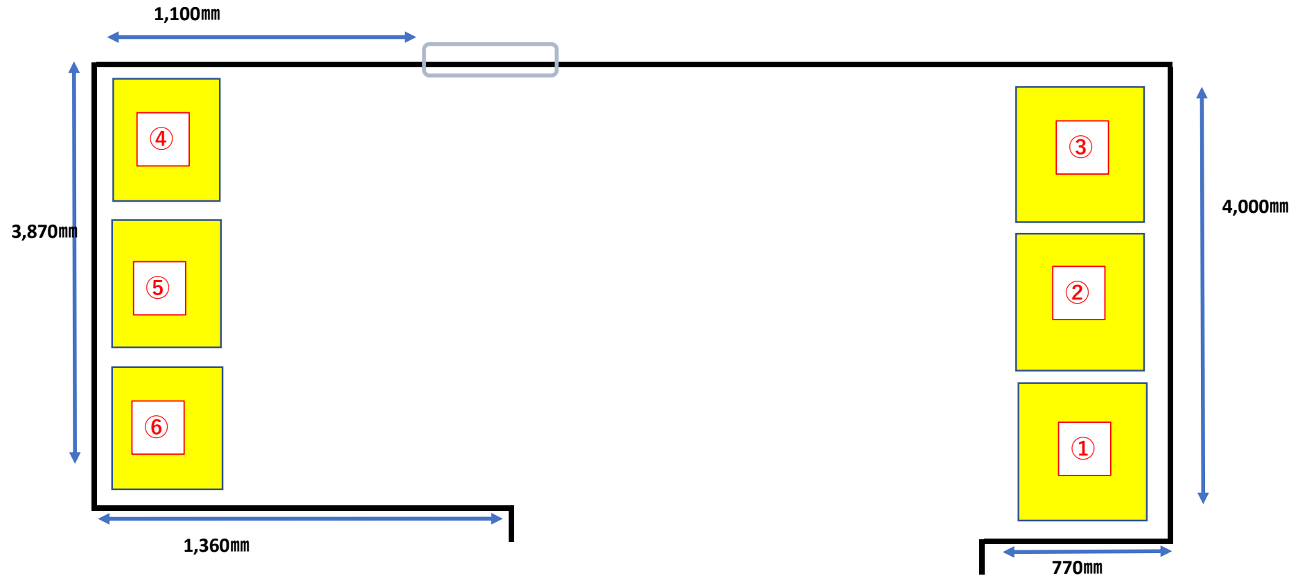
設置図
