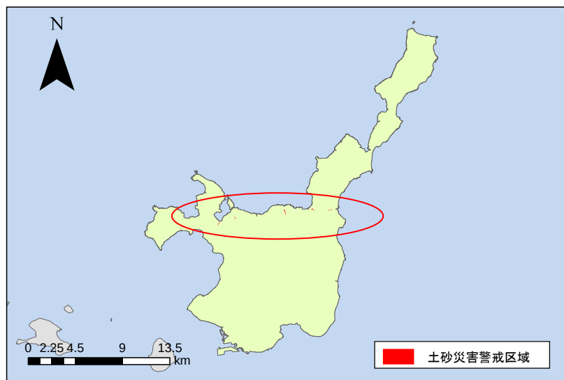
図 3-16 土砂災害警戒区域
