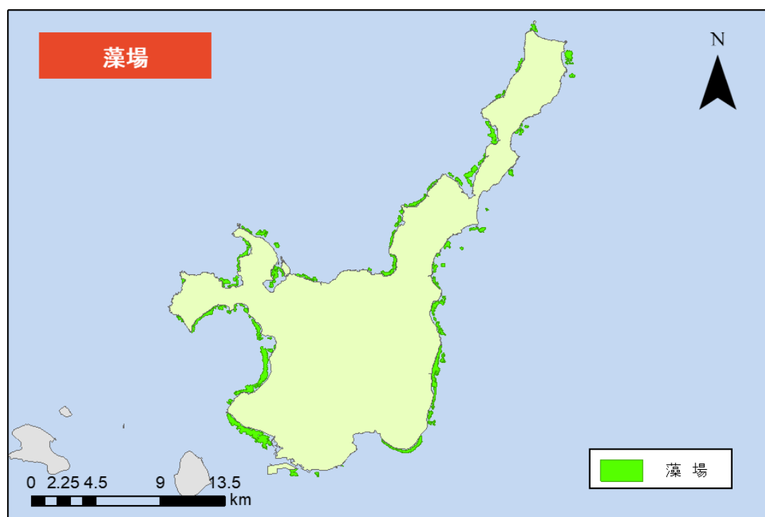
図 4-12 市域沿岸の藻場の分布状況
