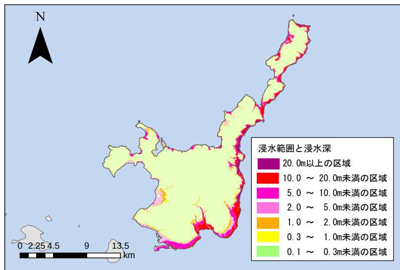
図 3-18 津波浸水想定区域・浸水深
